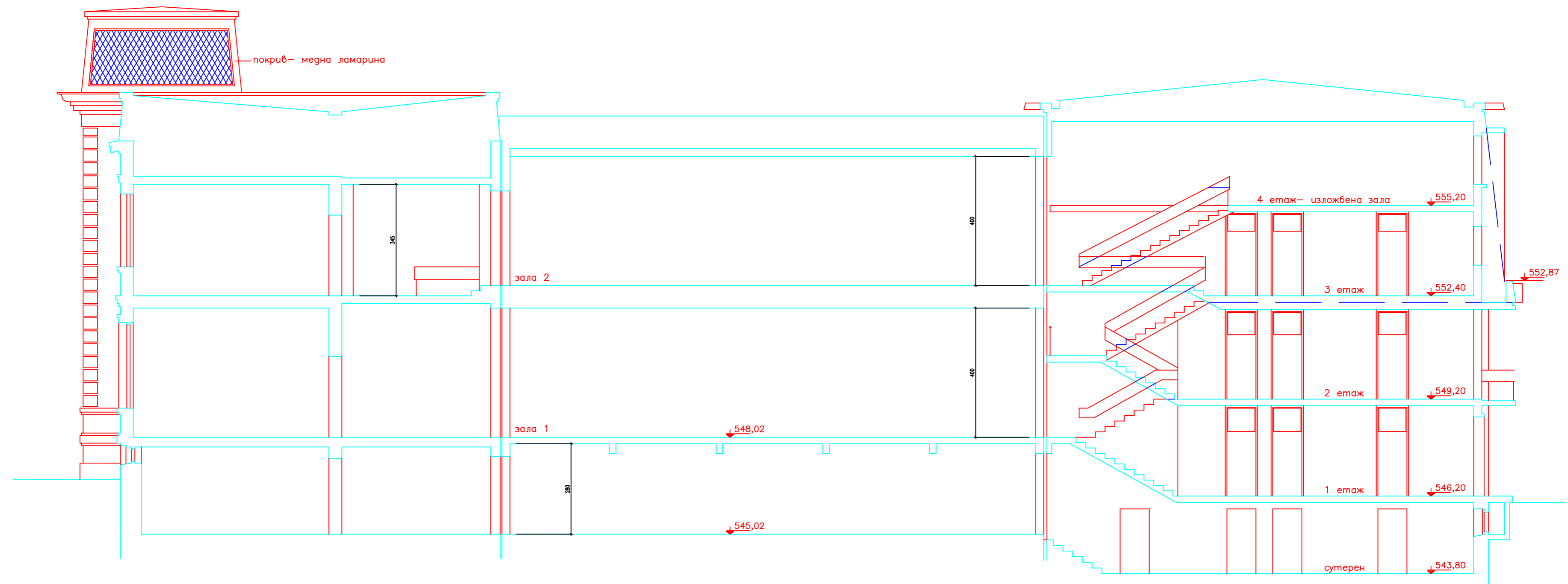
РАЗРЕЗ М1:50
